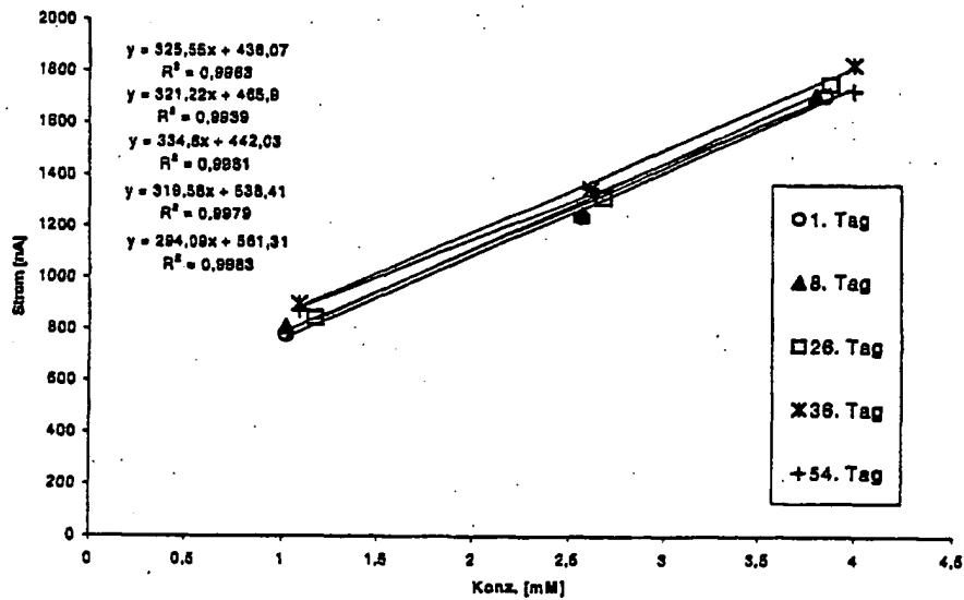
Abbildung 8: Sensitivität von ADPA-modifizierten Glukosebiosensoren mit PVP-Schutzschicht in Abhängigkeit des Sensoralters
